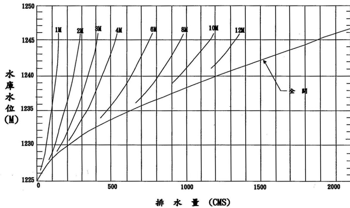
附圖一 青山壩排洪道率定曲線
