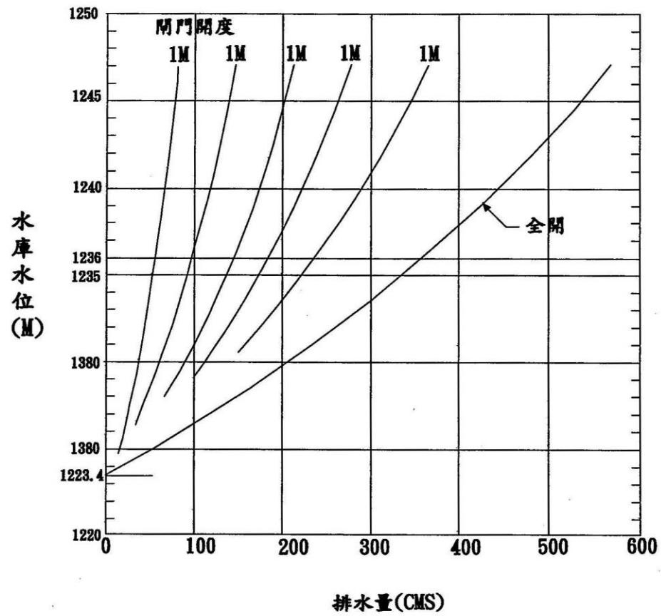
附圖二 青山壩排砂道率定曲線
